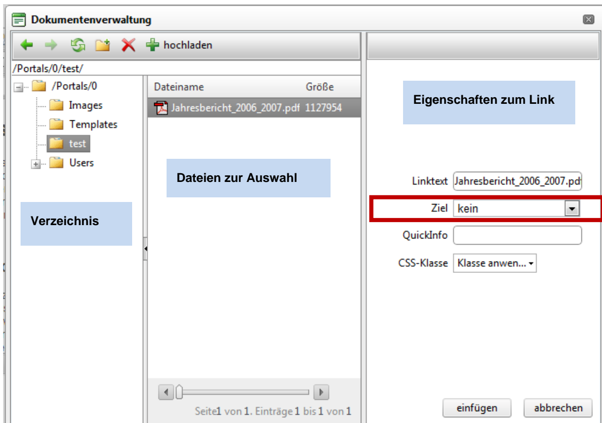
Abbildung 15: Dokumentverwaltung Ansicht
