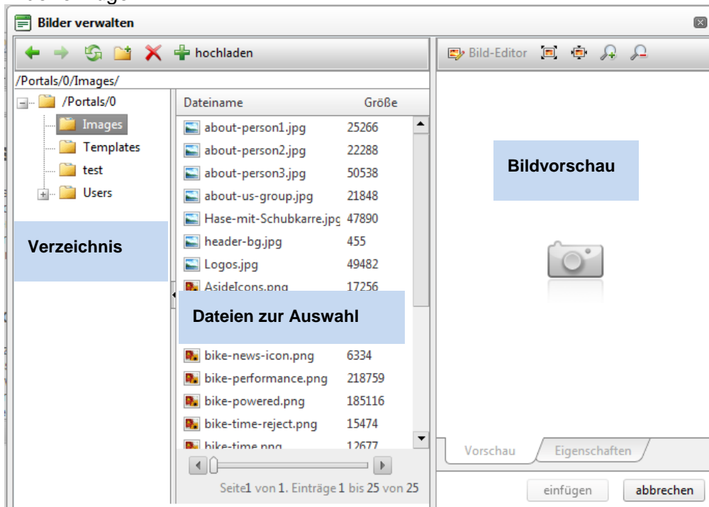
Abbildung 10: Bilder verwalten
