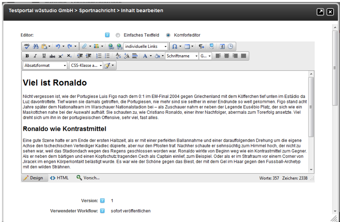
Abbildung 3: Inhalt bearbeiten
