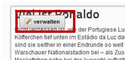
Abbildung 1: Modul verwalten
